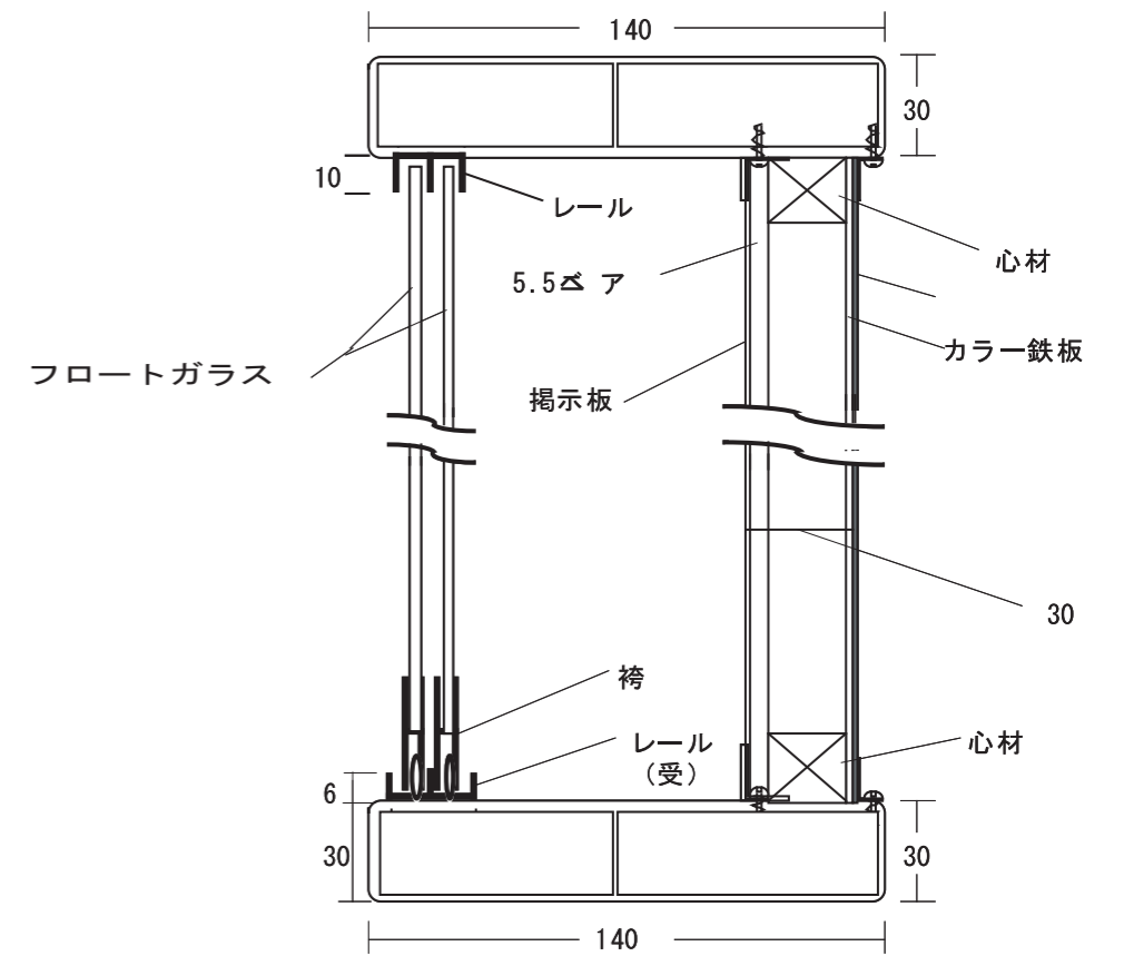
断面図
